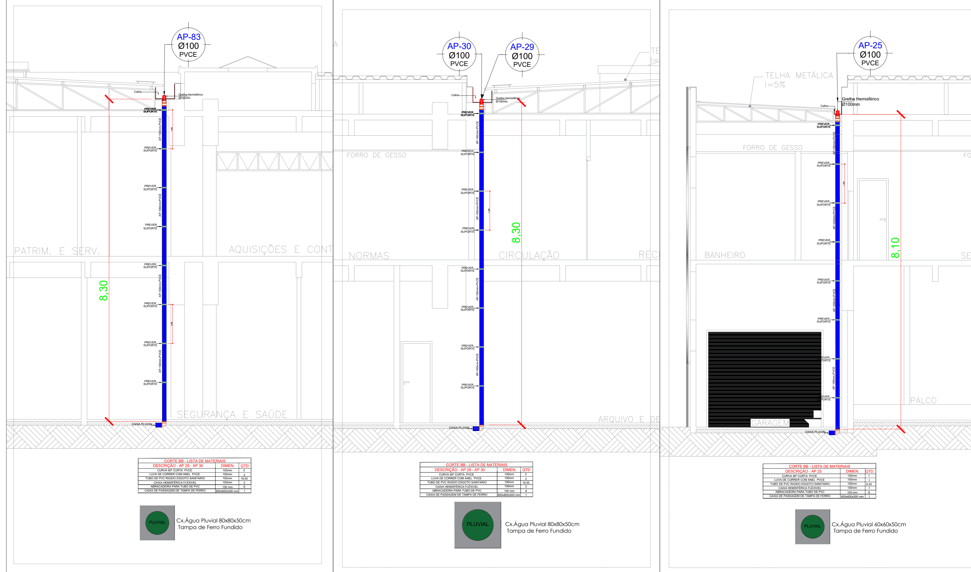
DETALHE - COLUNA AP-83 ESCALA: 1:50
