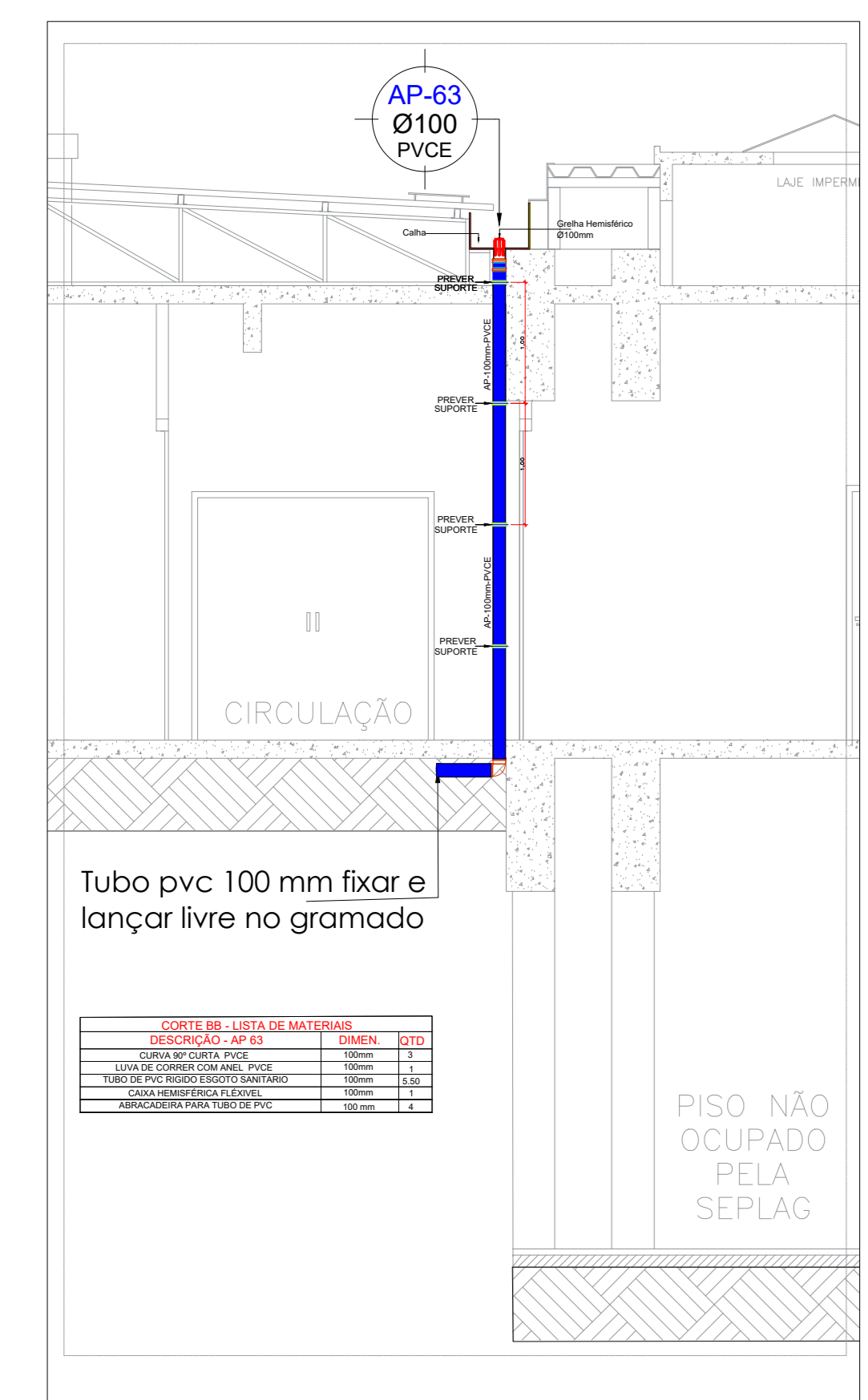
DETALHE - COLUNA AP-63 ESCALA: 1:50
